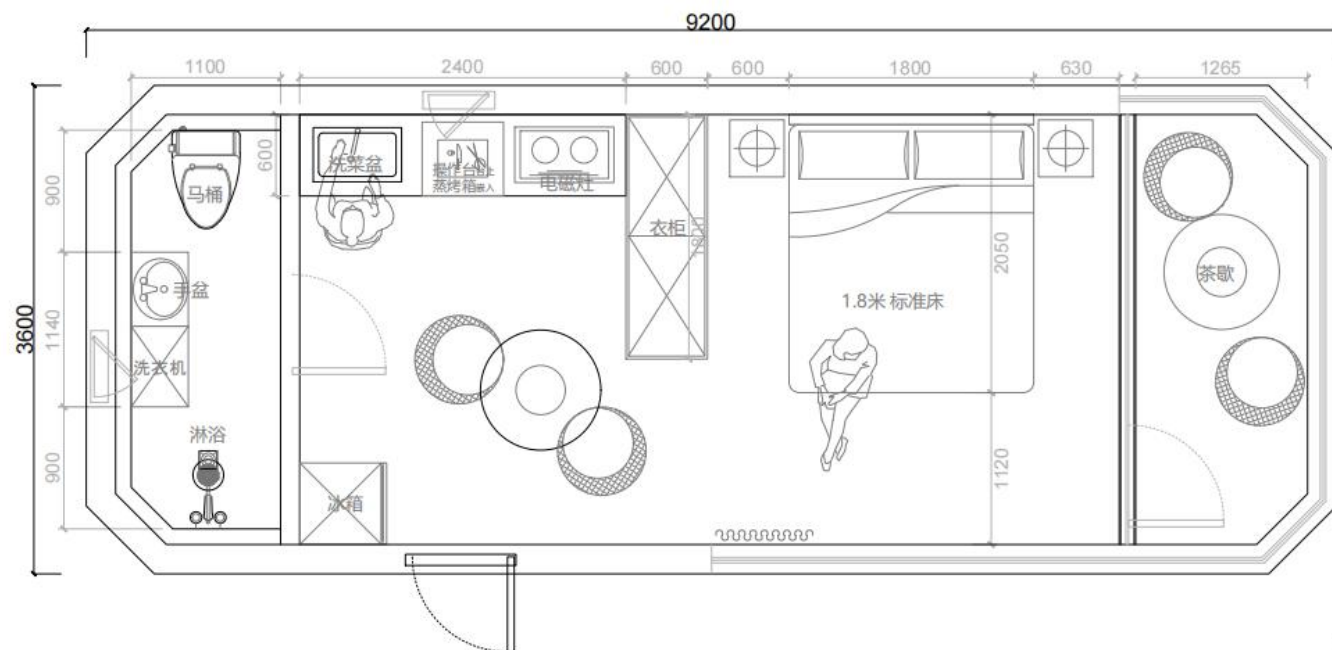
摩椅座-9200
