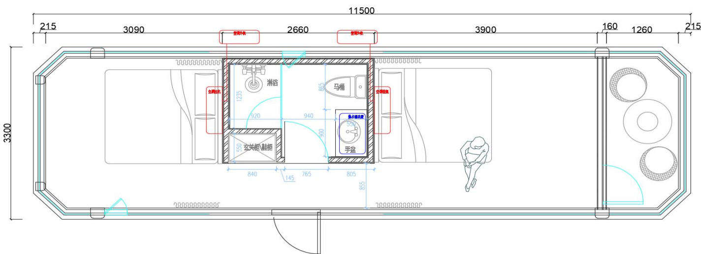
S70 平面布局
