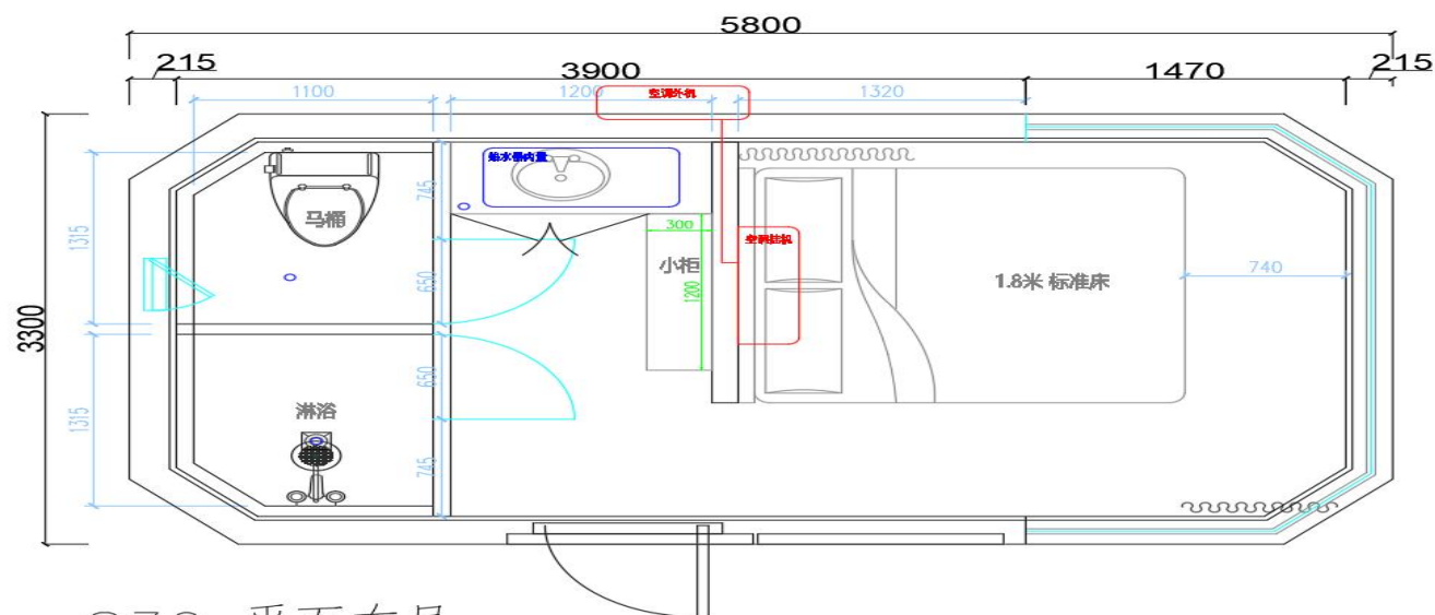
S30 平面布局
